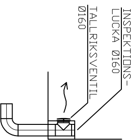
DETALJ 2-2 UTELUFTSDON VID GOLV A3/1:50
