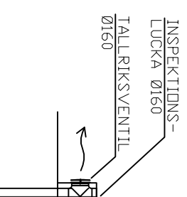
DETAIL J 2-2 UTELUFTSDON VID GOLV A3/1:50
